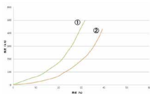
ロープ径60mmの強伸度曲線
